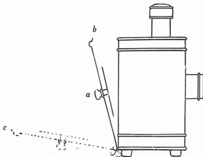
Darstellung der Türe und des drehbaren Bildhalters. (D. R. G. M. und D. R. P.).
