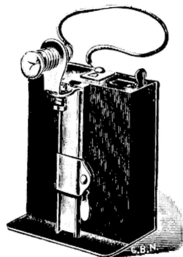
Lampe électrique avec pile sèche pour éclairage de petits cinémas à lanterne magique.
